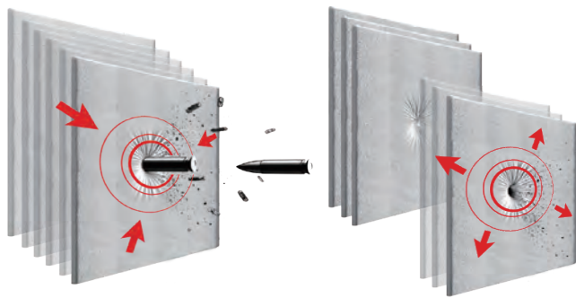
第1時間 衝擊UD布受力 第2時間 UD布能量傳播
